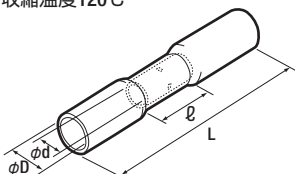
パーツ寸法
