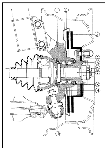
ブレーキローターのハット内側に ハブが装着されているタイプ （ホイールと共締めるタイプ）
