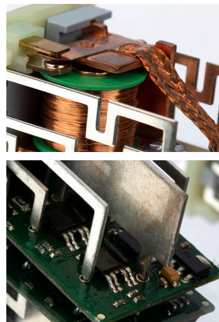
Relè meccanico originale della candele (in alto) rispetto ai semiconduttori intelligenti Astemo n. 2502183 (in basso)
